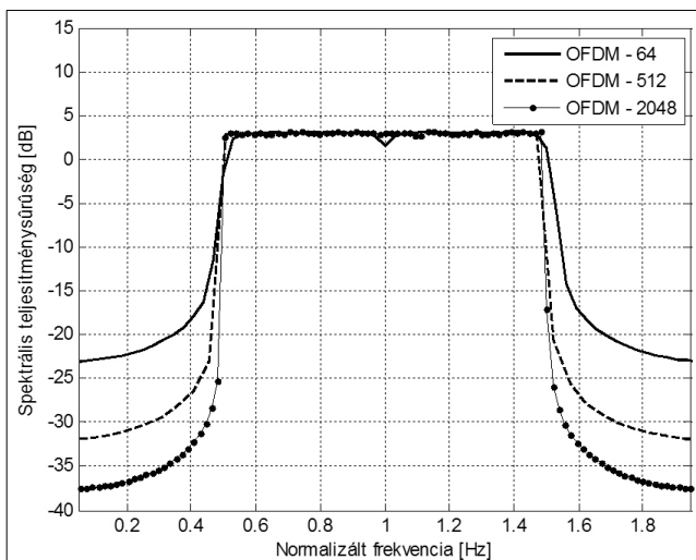
2. ábra Az OFDM rendszer spektrális sűrűsége
