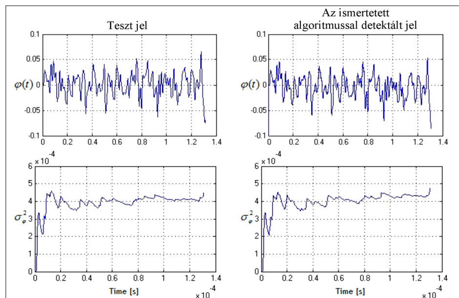
4. ábra A bemenő és a kinyert fáziszaj összehasonlítása. A \sigma_{\varphi}^2 variancia nem függ az időtől, az ábra azt mutatja, hogy a Simulink hogyan közelítette az idő függvényében
