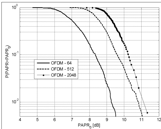
3. ábra A csúcstényező eloszlásfüggvénye
